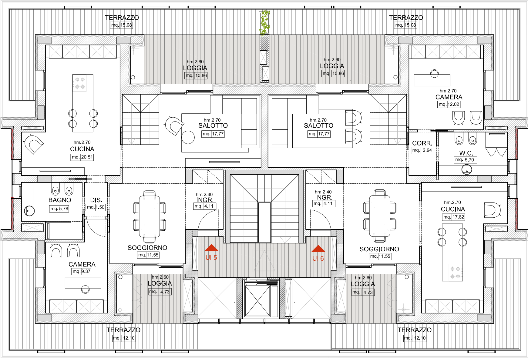
Pianta Piano Secondo sc.1:100
