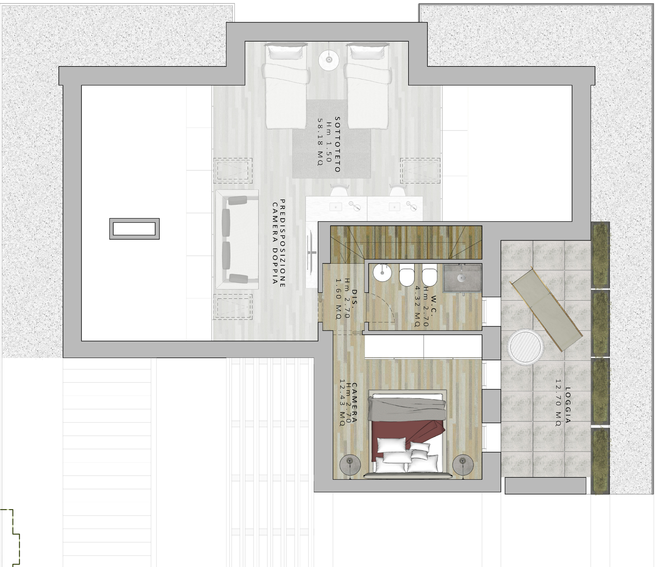
Tipologia U5/6 sc1:50
